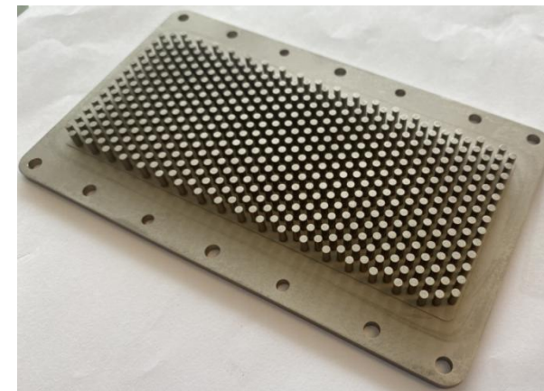
銅/鋁散熱片
